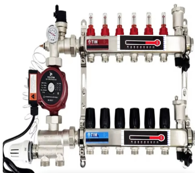
Razvodnik za podno grejanje
